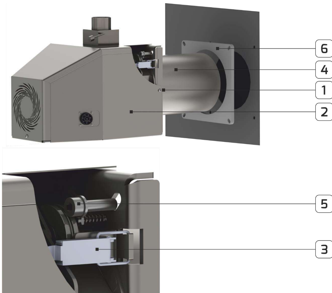
Рис. 9. Монтаж модели от REVO 44 до REVO 150 в дверце котла.
