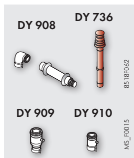
Горизонтальное окончание из алюминия для коаксиального дымохода, Ø 60/100 мм
