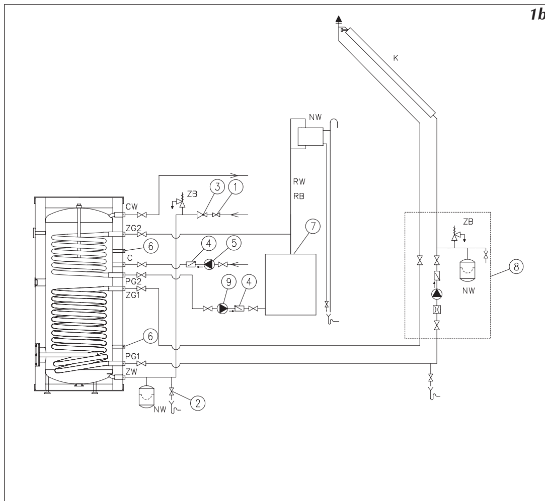
Рис.1b Схема подключения теплообменника с системой солнечной водонагревательной установки и отопительным твердотопливным котлом, система защищена согласно обязывающим нормам -система открытого типа
