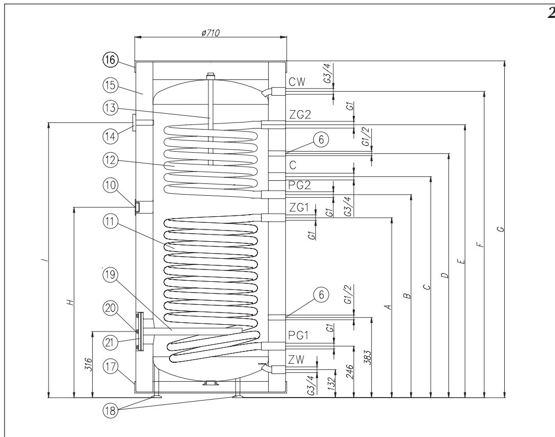
Рис.2 Конструкция теплообменника SB
