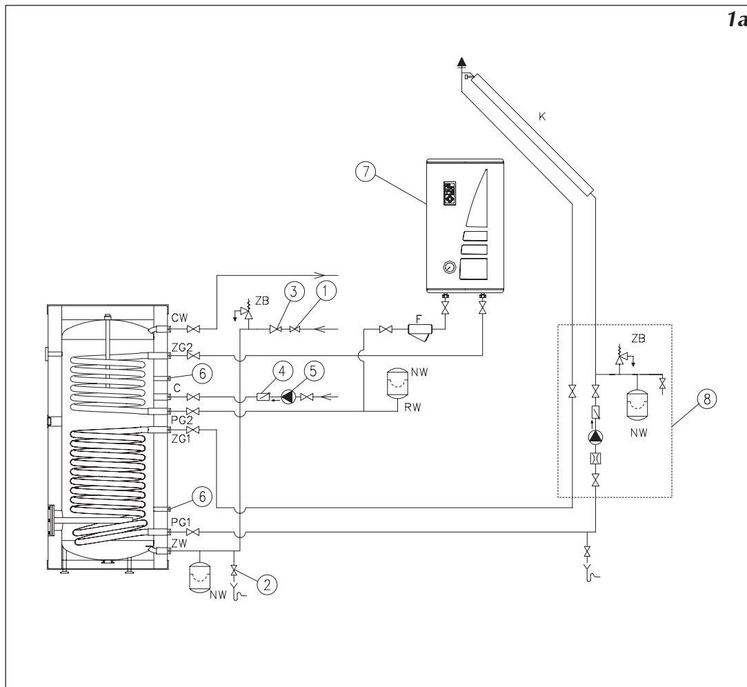
Рис.1а Схема подключения теплообменника с системой солнечной водонагревательной установки и отопительным котлом (электрическим, газовым, жидкотопливным), система защищена согласно обязывающим нормам – закрытая система.
