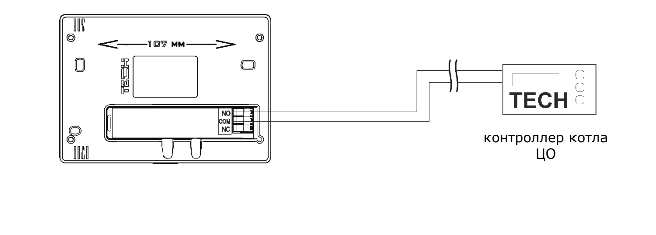
2 Схема подключения регулятора ST-290 с контроллером котла ЦО.
