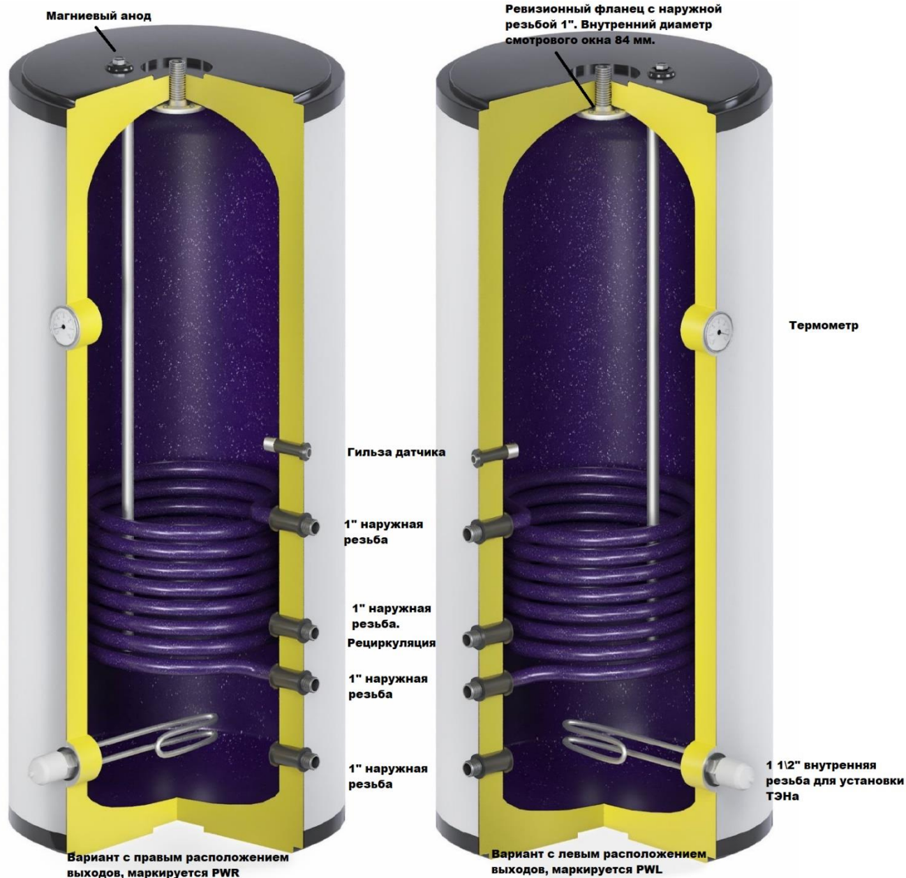
PWR- с правым подключением
